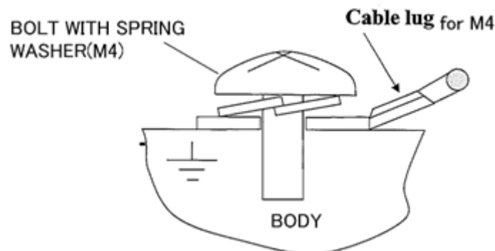
그림 3 케이블 러그
